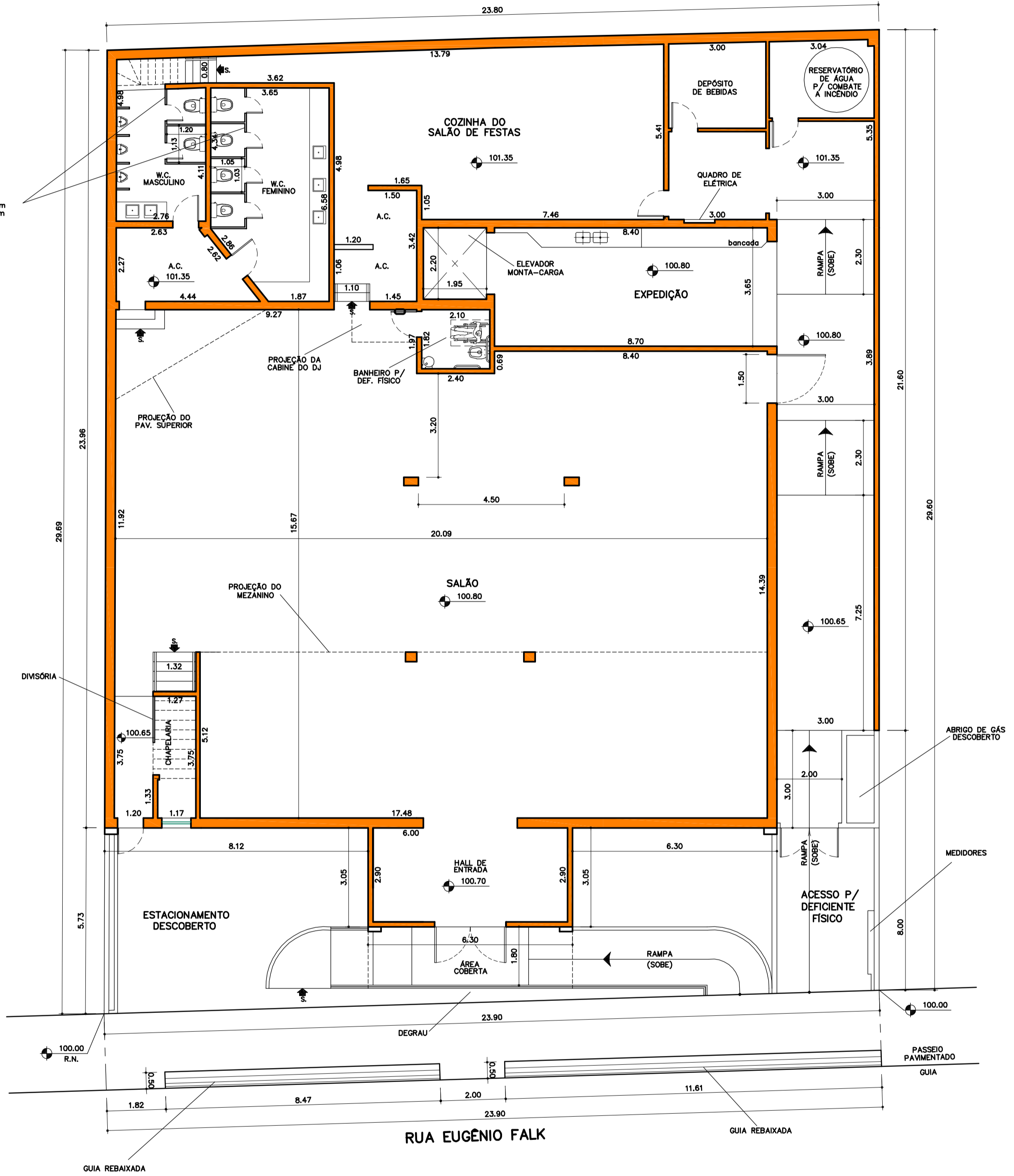
PLANTA DO PAV. TÉRREO (ESC.1:100)
